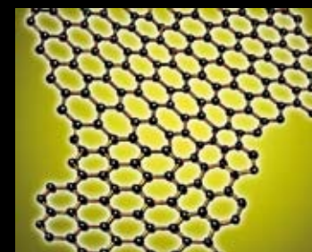
Grafeenstructuur
